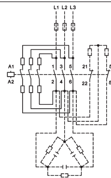
Schaltbild für Anschluß von Schnellentladewiderständen
