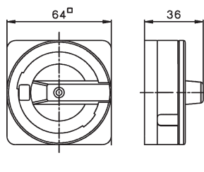
Sperrvorrichtung SV4
