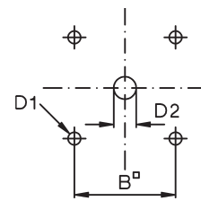
Bohrplan: TKZ
