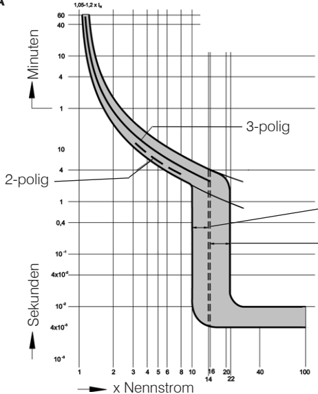
0,16 - 16A
