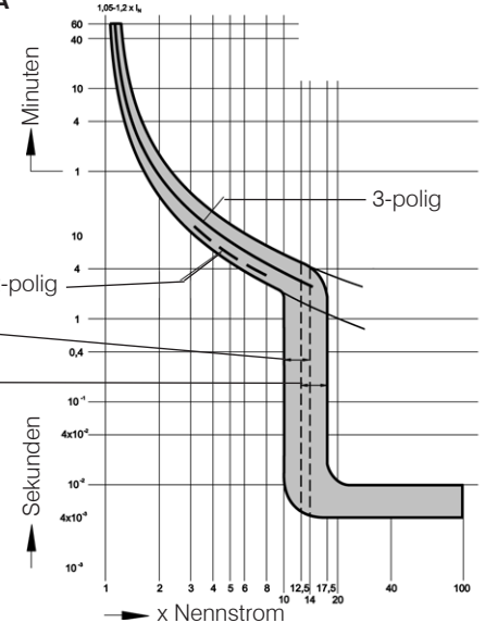
16 - 32A
